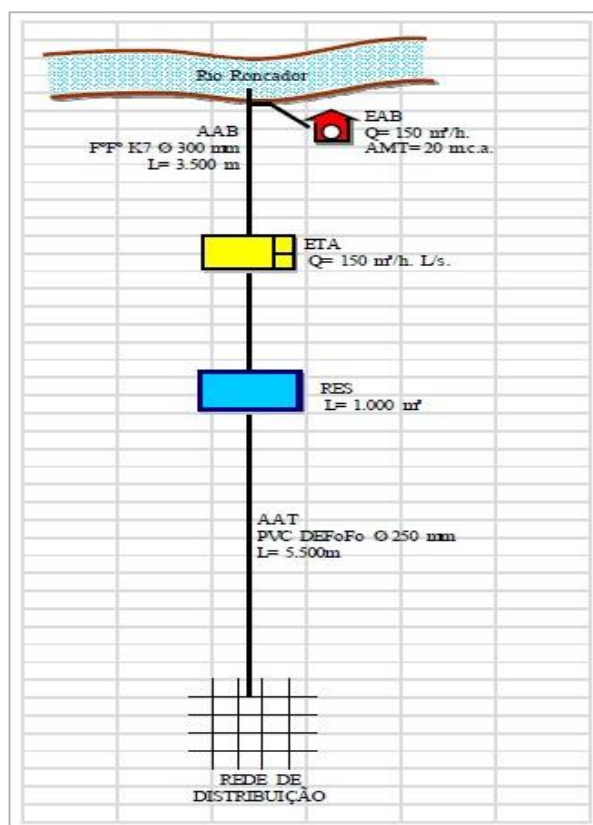
Figura 9: Diagrama simplificado do SAA Jaconé, distrito de Sampaio Correia
